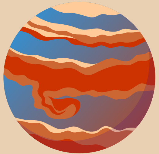
JUPITER
