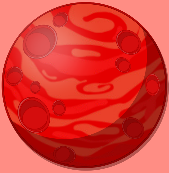
MARTE
