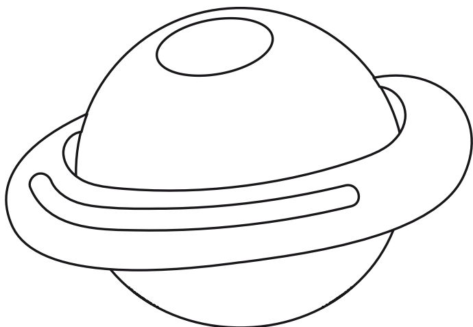
SATURNO
