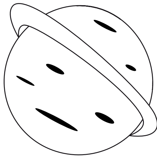
URANO
