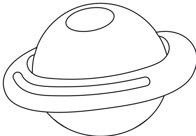
SATURNO
