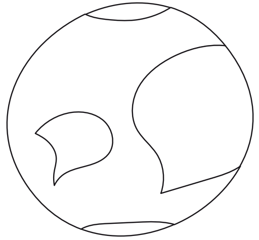
MERKURIO
