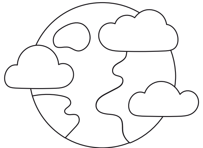
LURRA
