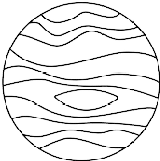
JUPITER
