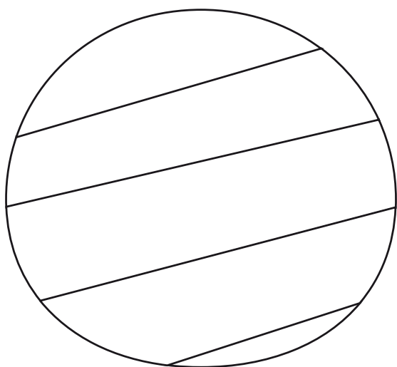
NEPTUNO
