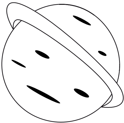
URANO
