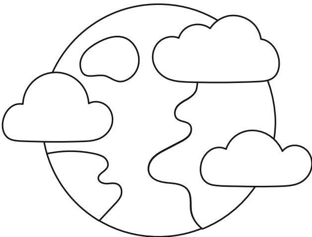
LURRA
