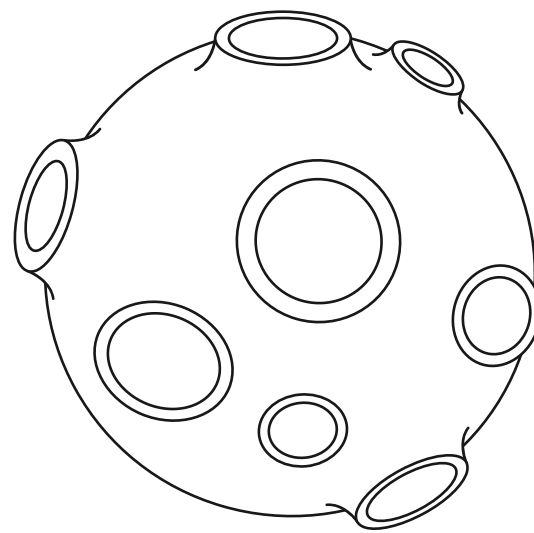
MARTE
