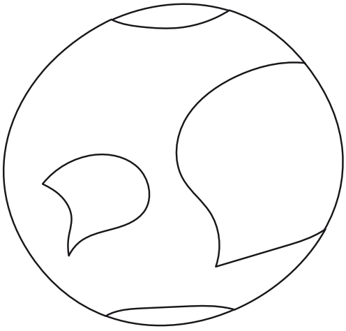
MERKURIO
